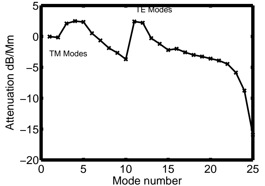
Attenuation factor shift
