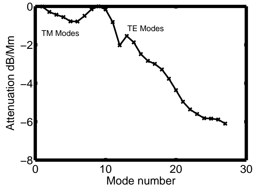
Attenuation factor shift
