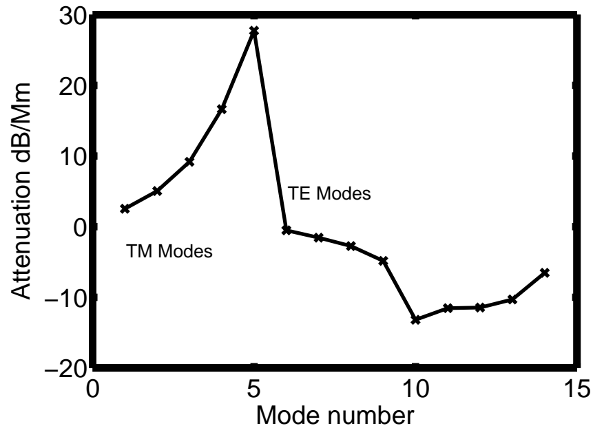
Attenuation factor shift
