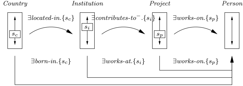
Fig. 6. mSpace example
