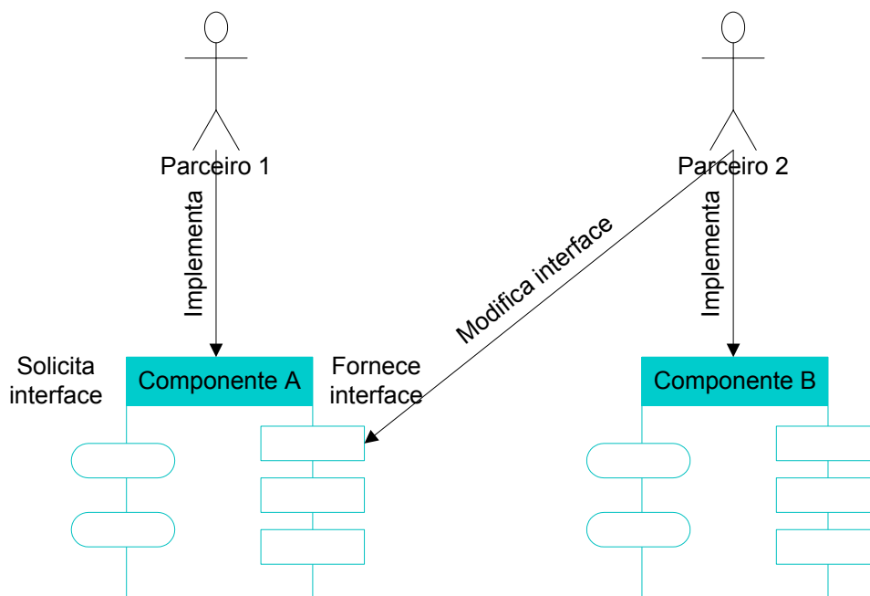
Figura 5 – Mudança de interface de componente
