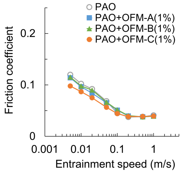
(d) steel-steel (50% SRR)
