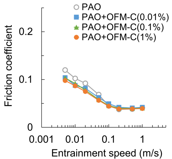
(d) steel-steel (50% SRR)
